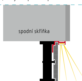
b) uchycení pro LED profil
