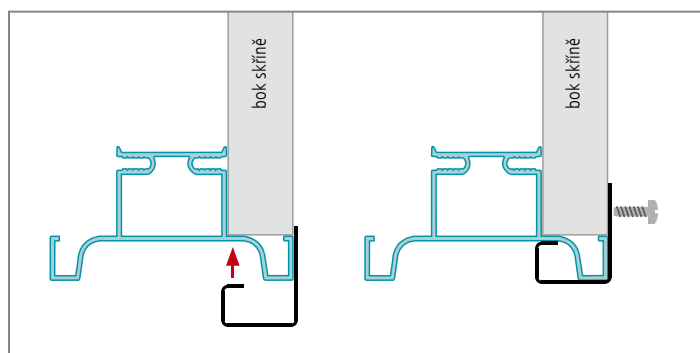
Montáž profilu S044 s profilem S059
