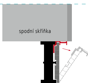
a) demontáž soklu
