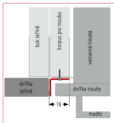
Umístění boční ochranné lišty MT/bocni (levá strana, pohled shora)
