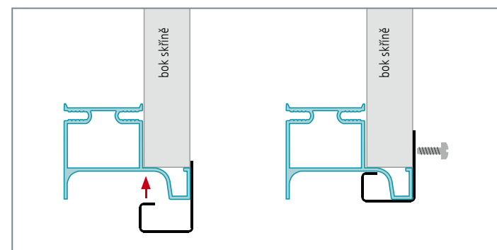
Montáž profilu S044 s profilem S060
